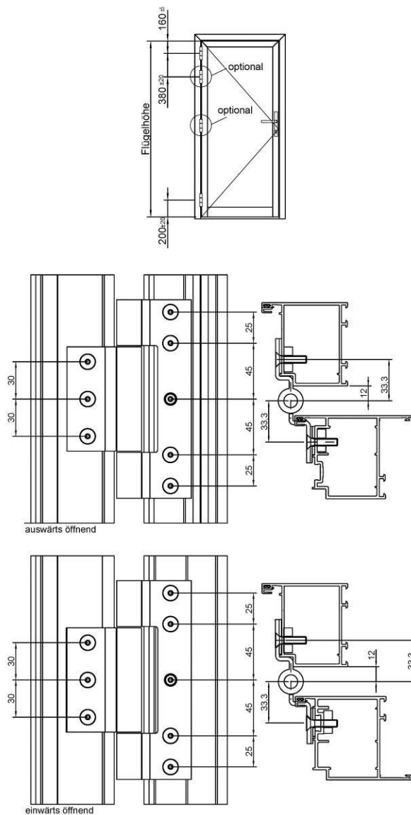
Rollenband ECO
